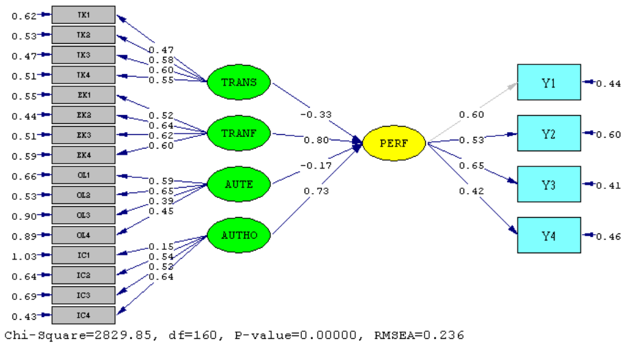
Gambar 2 Memuat Nilai Indikator Catatan : Gambar berasal dari proses output program Lisrel
